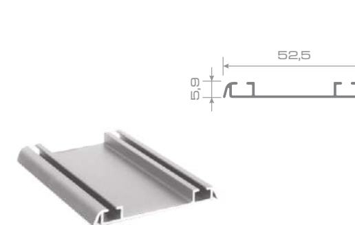
ТРЕК НИЖНИЙ ЛАЙТ
