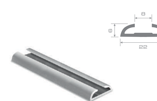
ТРЕК ДЛЯ РАСПАШНОЙ ДВЕРИ
