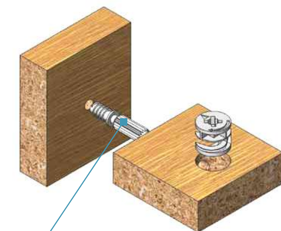
ШТОК ЭКСЦЕНТРИКОВОЙ СТЯЖКИ
